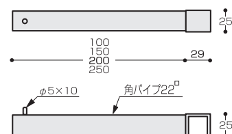
OFSS-22 □ シングル
