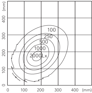
45°首振り時水平面照度 (H200mm) Horizontal illuminance when down 45° neck(H200mm)
