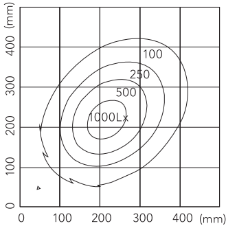
45°首振り時水平面照度 (H275mm) Horizontal illuminance when down 45° neck(H270mm)
