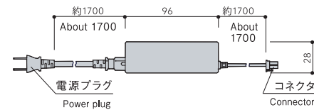
CNSA-96×44×28-2419
