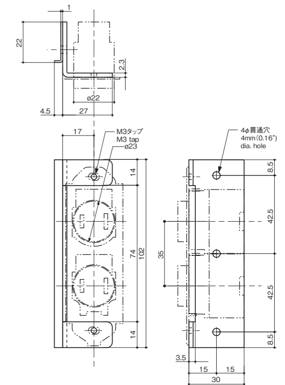
図面 ツインコンセント Drawing of the Twin Concent (WPC-22φW)
