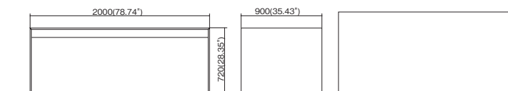
サイズ Size : W2000×D900×H720mm(78.74"×35.43"×28.35")
