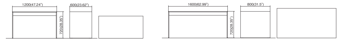
サイズ Size : W1200×D600×H720mm(47.24"×23.62"×28.35")
